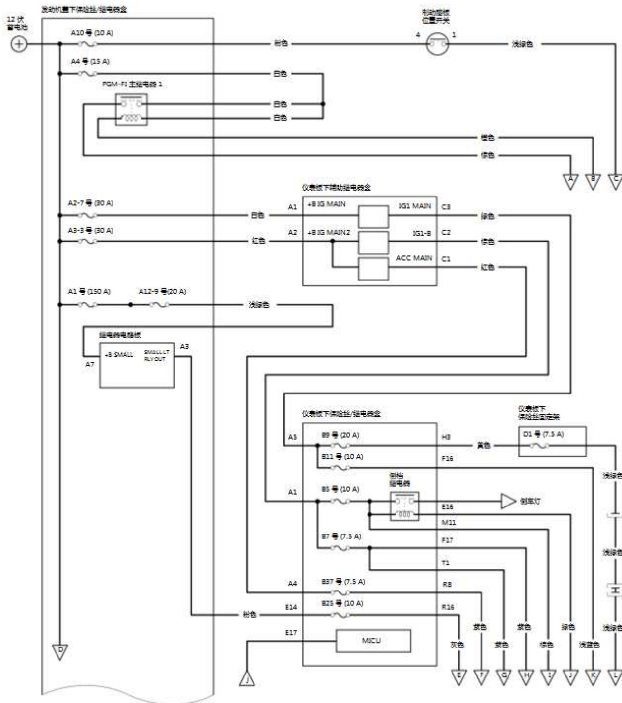
齿轮组控制系统电路图
